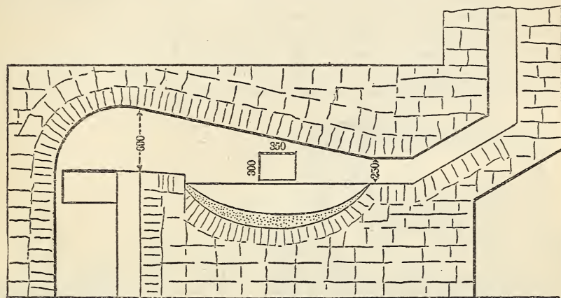
LONGITUDINAL SECTION.
